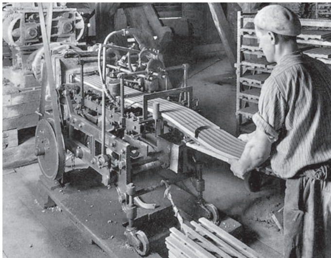
Früher wurden die Biberschwanzziegel mit solchen Strangpressen produziert und zum Trocknen auf Holzrähmchen gelegt.
